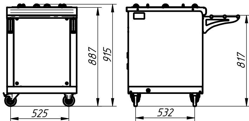
Вариант с поворотными колесами
